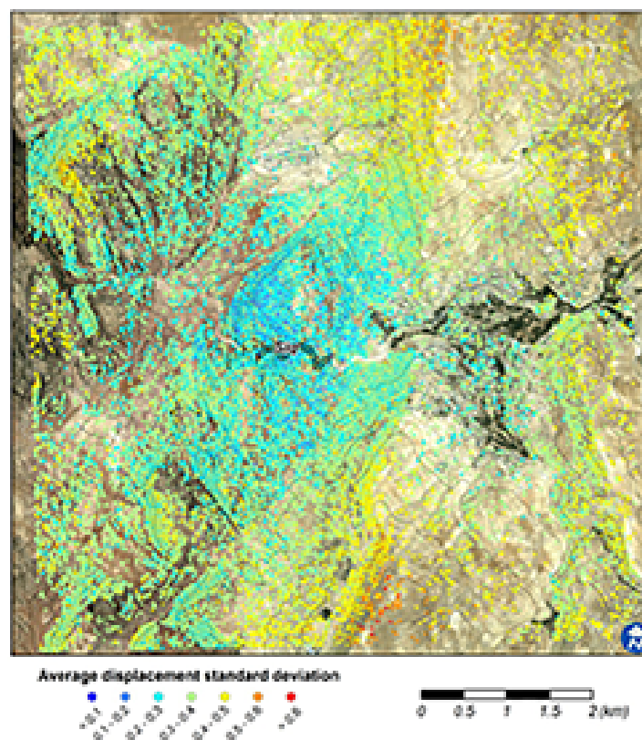
Fig. 1 Esempio di analisi interferometria per l'individuazione dei fenomeni deformativi e di instabilità geomorfologica nell'area di Petra in Giordania
