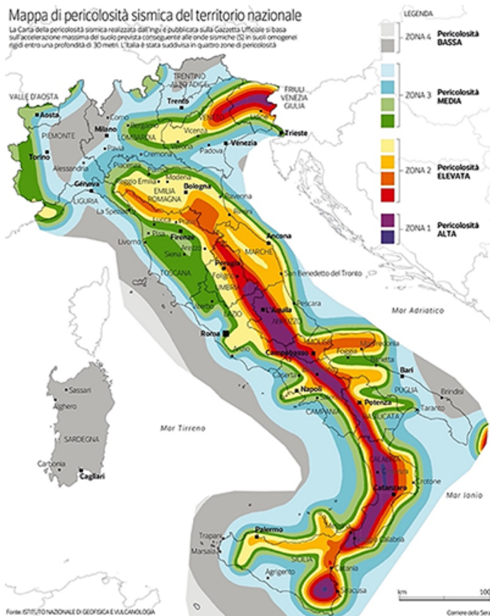
Fig. 5 Mappa di pericolosità sismica del territorio nazionale denominata MPS04, perché completata nella primavera del 2004 ( http://zonesismiche.mi.ingv.it/ ), ridisegnata dal Corriere della Sera. I colori mostrano i diversi valori di PGA che hanno una probabilità del 10% di essere superati in 50 anni. La mappa è alla base della vigente normativa antisismica italiana, riassunta nelle Norme Tecniche per le Costruzioni varate nel 2008 (NTC08) e aggiornate nel 2018 (NTC18)
