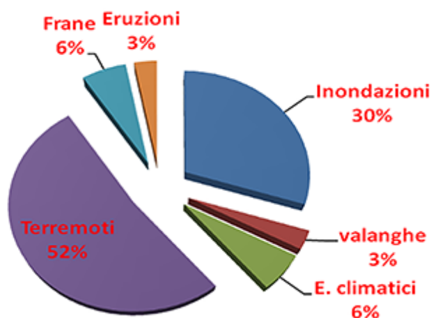
Fig. 12 Numero di vittime in Italia in base alle tipologie di eventi estremi dal XX secolo
